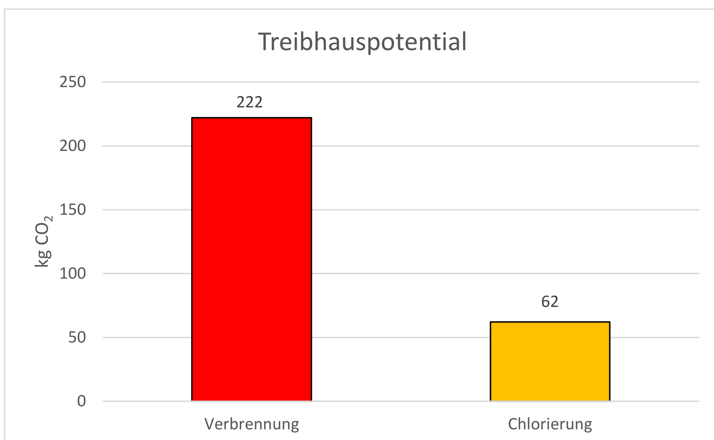
Abbildung 1: Treibhauspotential für die Chlorierung und Verbrennung von einer Tonne LCD-Panels.
