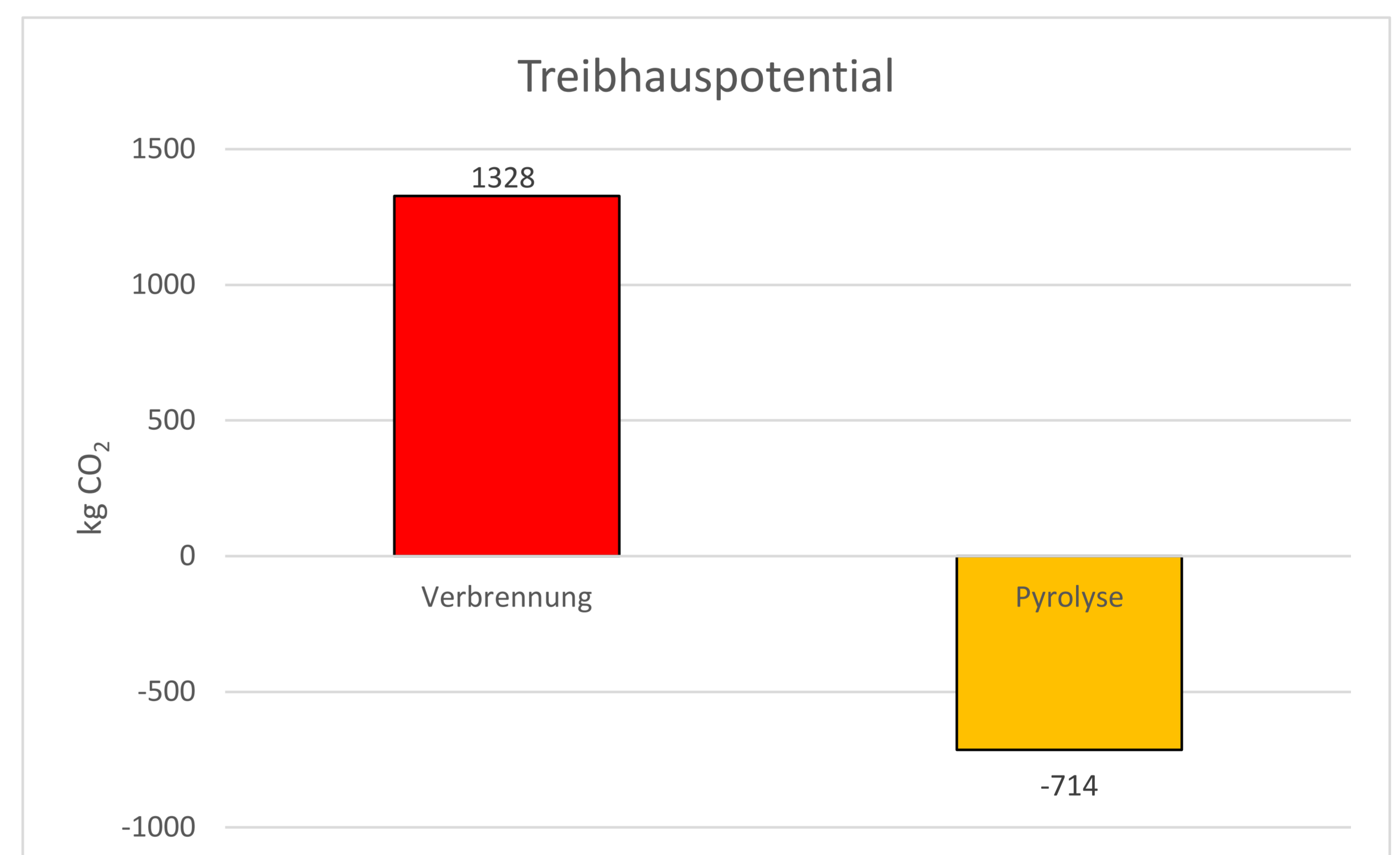
Abbildung 2: Treibhauspotential für die Pyrolyse und Verbrennung von einer Tonne PVC-Abfälle (ca. 50% Chlorgehalt).
